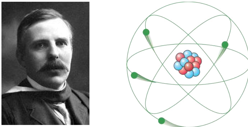
Figura 1.9. Izquierda: Ernest Rutherford. Derecha: Modelo atómico de Rutherford. El núcleo contiene los protones y neutrones; los electrones orbitan el núcleo, en similitud al sistema planetario.
