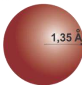
Figura 2.4: Diferencia entre el radio atómico del Bario (izquierda) y el ión bario (derecha). En los cationes, el radio iónico es siempre menor al radio atómico; por el contrario, en los aniones, donde el ión adquiere carga negativa, el átomo incrementa en tamaño, por lo que el radio atómico de un anión es siempre mayor que el del átomo neutro.
