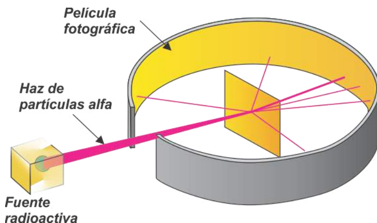
Figura 1.7. Experimento de Rutherford. Una fuente de partículas alfa ingresa en un cilindro cubierto internamente por una placa fotográfica sensible a las partículas radioactivas; al alcanzar una delgada lámina de oro, el modelo de Thomson permite predecir que la gran mayoría de los haces atravesarán la lámina metálica, y solo una fracción de la radiación atravesada sufrirá desviaciones menores.
